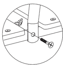
Рис.3 Крепление спинки
