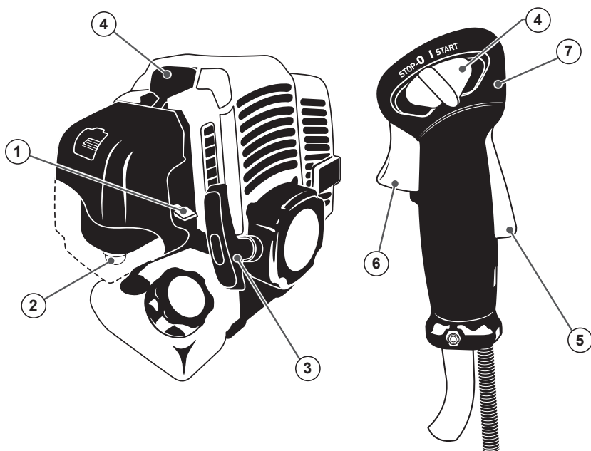
Рис. 7. Органы управления
