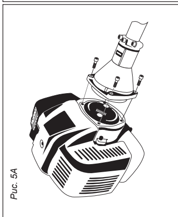
Рис. 5. Схема сборки
